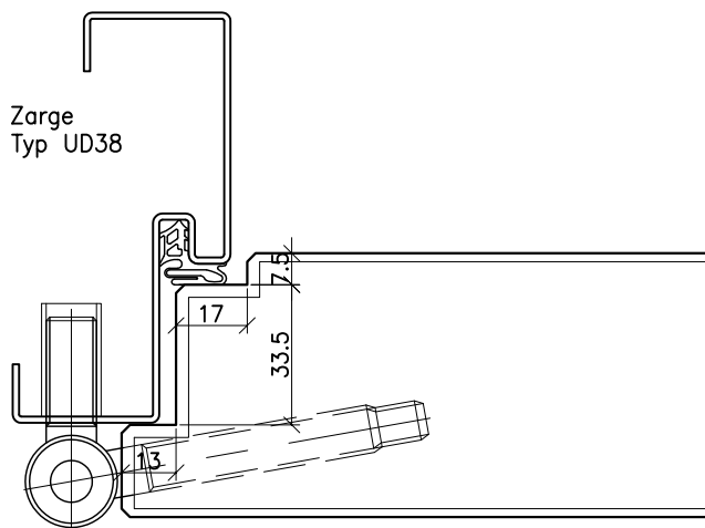
Zargenband HE22
