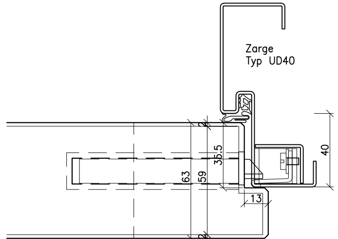
Glutz 1106 RZ
