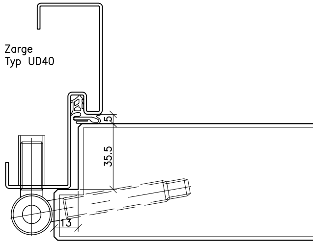
Zargenband HE22
