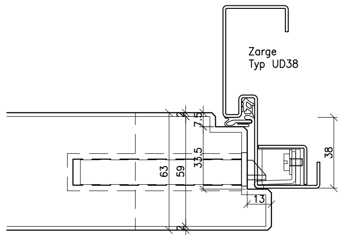
Glutz 1106 RZ
